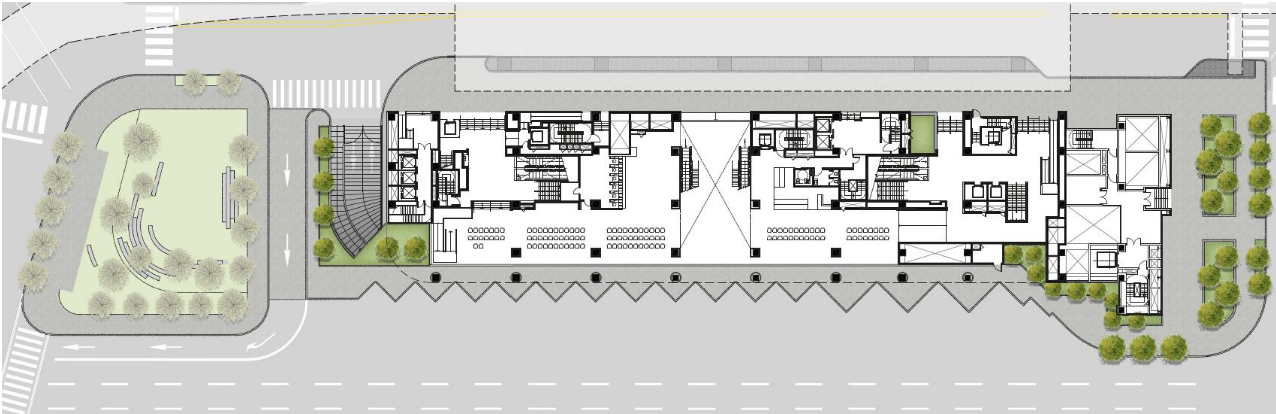
一層平面圖
